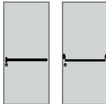
Greep met drukknop | Bar with push button
