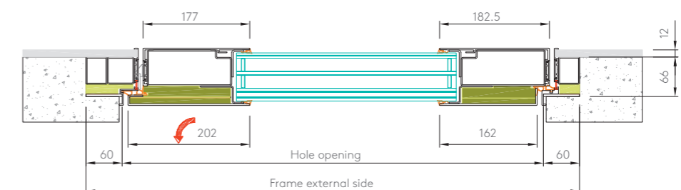
Deur bovenaanzicht trekversie - Door horizontal section with pull opening
