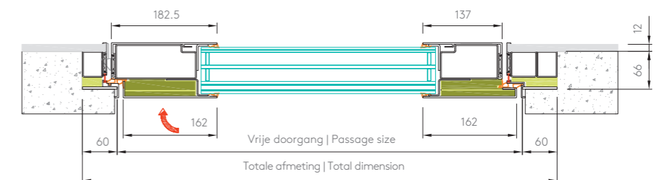
Deur bovenaanzicht duwversie - Door horizontal section with push opening
