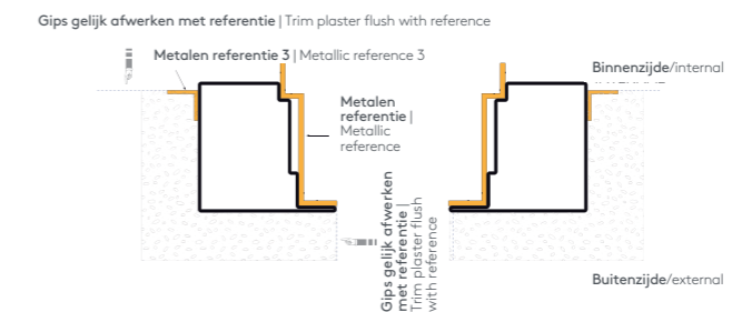
Vlak met Boiserie aan de binnenzijde Flush with internal wall with Boiserie
