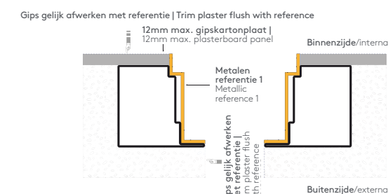
Vlak met binnenwand met gipskarton Flush with internal wall with plasterboard
