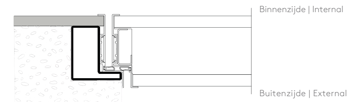
Vlak met buitenwand | Flush with external wall
