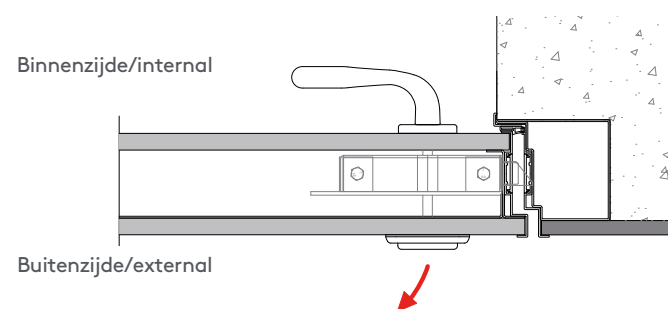
Deur bovenaanzicht trekversie - Door horizontal section with pull opening
